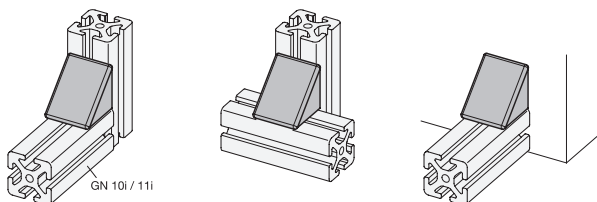
Przykład montażu
